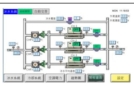
銓冠-富強醫材
