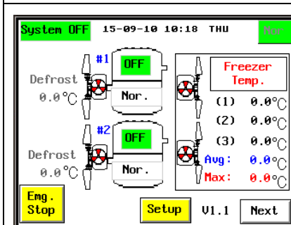
吉昌_喜康生冷凍庫
