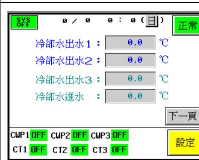
清華大學水冷直膨系統
