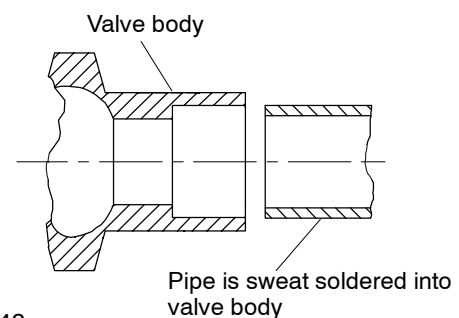
Fig. 26. 3/4" Sweat
