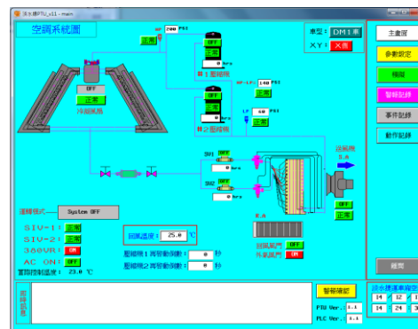
捷運車廂 381 空調系統-整改前
