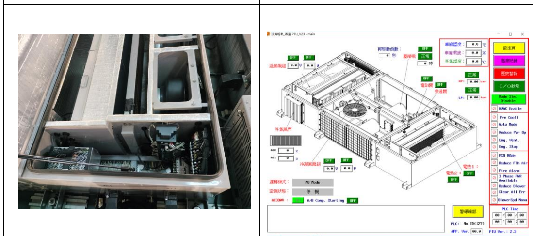
安坑輕軌車廂空調系統
